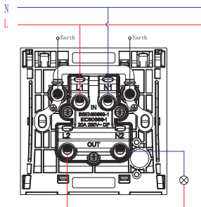
1G switch 20A DP
