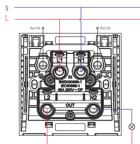
1G 45A switch DP
