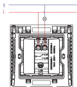
1G 1W switch
